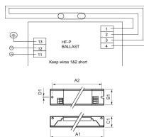
Scheda tecnica Philips HF-P 1 14-35 TL5 HE III 220-240V para 1x14-35W Fluorescente
